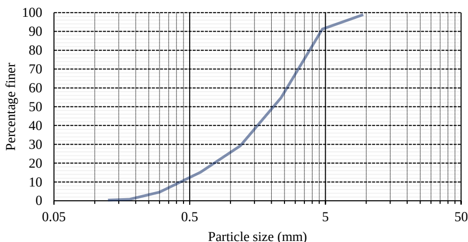
شکل ۱. منحنی دانه‌بندی سنگ‌دانه‌ها
