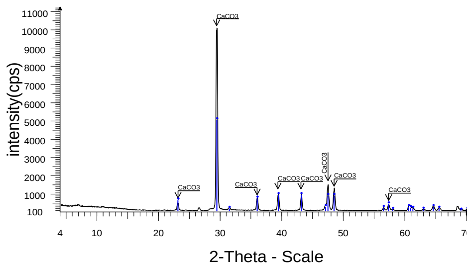
شکل ۴. نتایج حاصل از XRD نانوکلسیت
