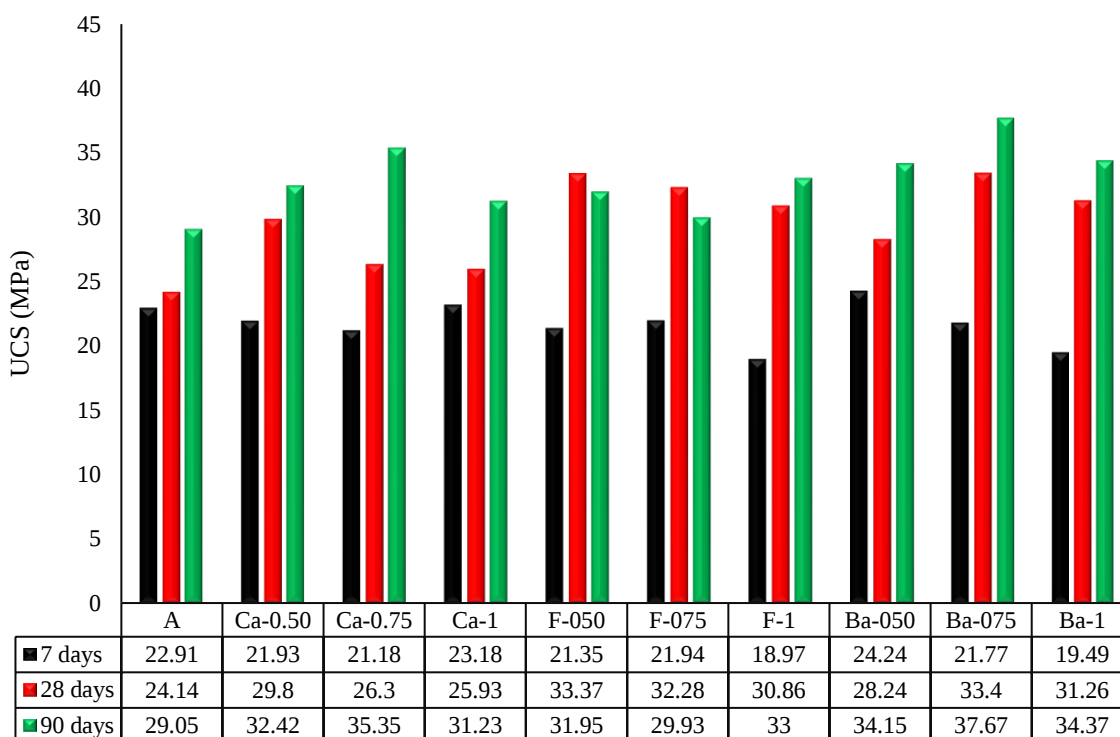
شکل ۱۹. مقایسه مقاومت فشاری نمونه‌ها با یکدیگر
