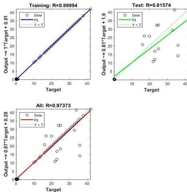
شکل ۱۲. نمودارهای شبکه‌ی عصبی q
