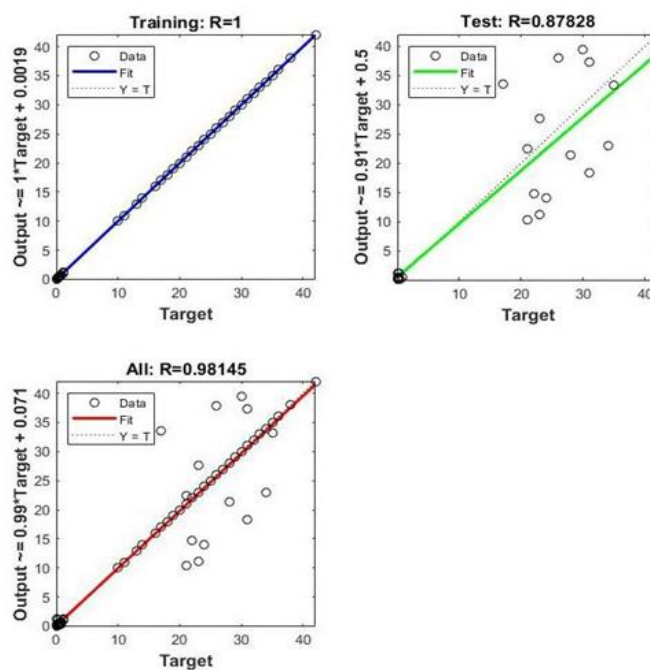
شکل ۱۱. نمودارهای شبکه‌ی عصبی P
