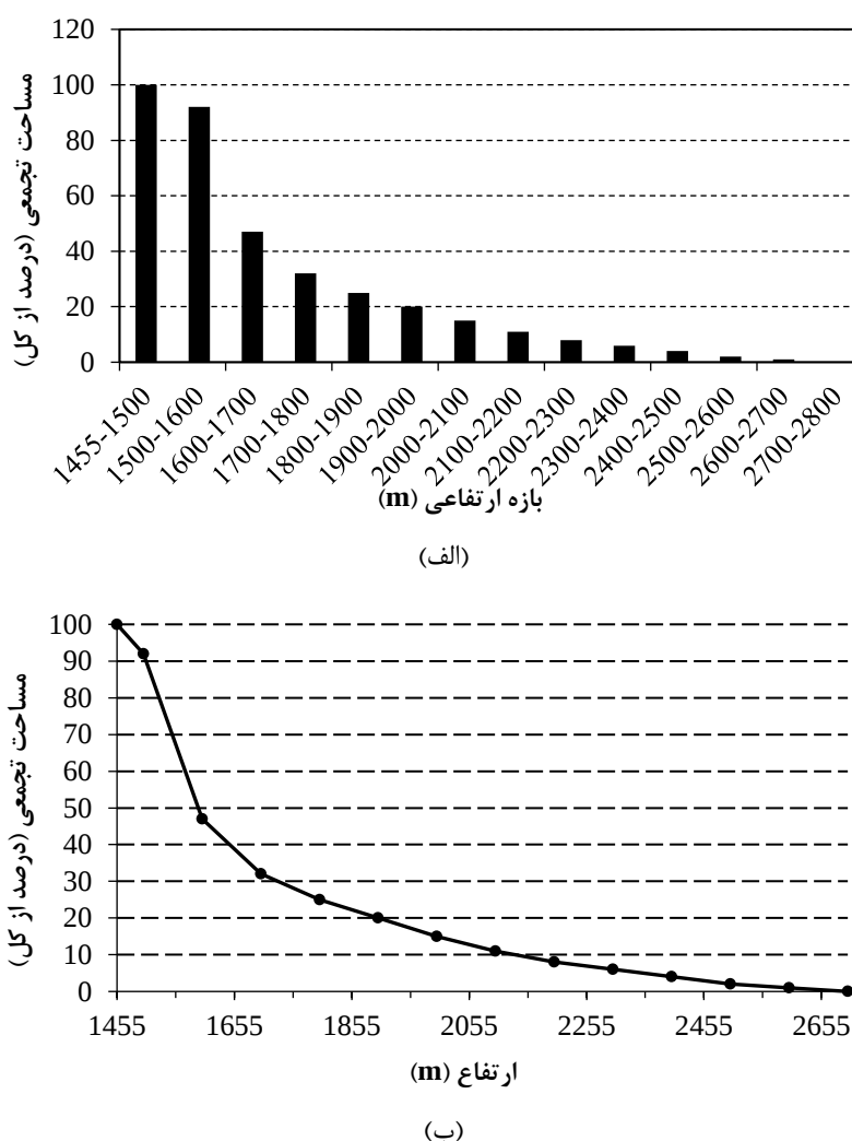
شکل ۷. نمودار توزیع تجمعی مساحت در ارتفاع برای حوزه آبریز رودخانه گیان
