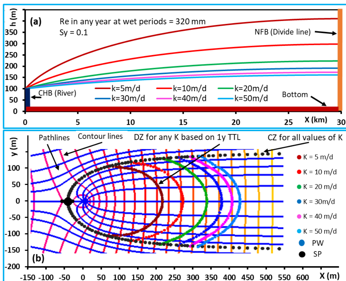
شکل ۵. اثر هدایت هیدرولیکی (K): (a) سطح آب نرمال در پایان دوره‌ی تر. (b) حریم آگیر و حریم تخلیه. خطوط زمان گذر یک ساله هستند.
