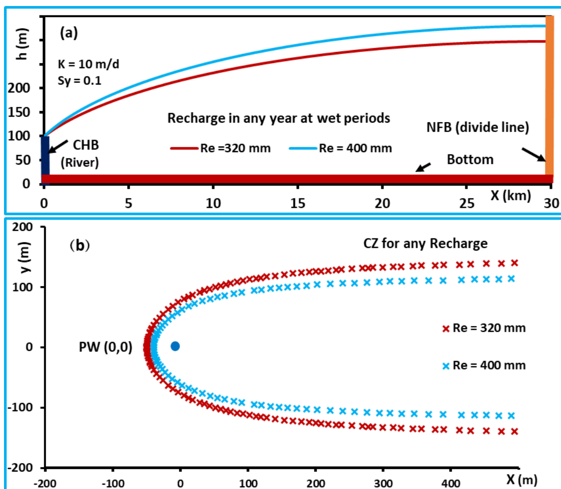
شکل ۱۵. اثر نسبت تخلیه به تغذیه بر حریم آگیر در چاه مرکزی آبخوان. شکل تغییر حریم آگیر چاهی در مرکز یک آبخوان را نشان می‌دهد که سطح تراز آن از طریق چاه‌هایی که به طور مناسب در کل آبخوان جانمایی شده‌اند تنزل یافته است. مقدار تخلیه‌ی کل چاه‌ها معادل ۸۰ میلی‌متر از کل تغذیه‌ی آبخوان بوده است.
