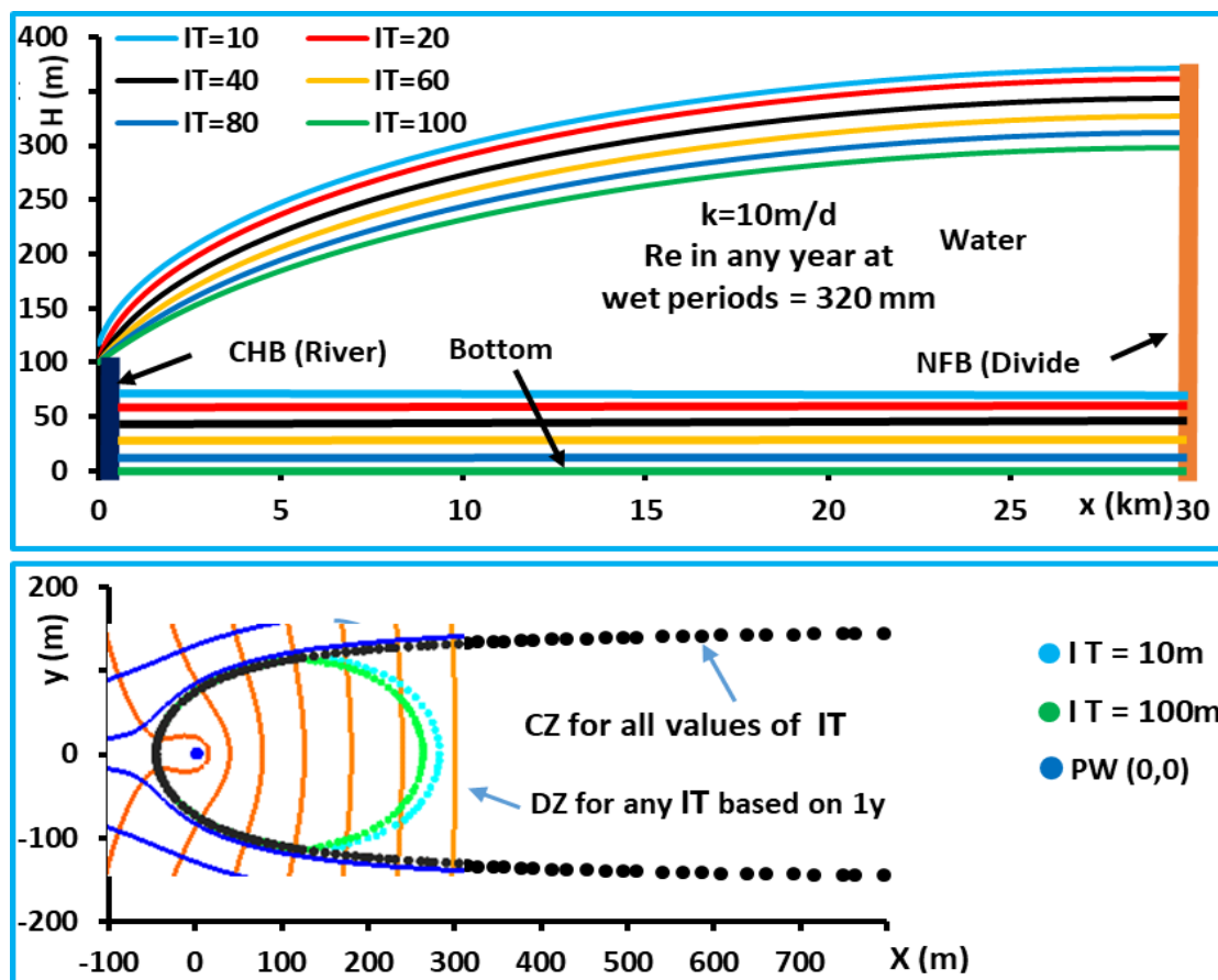
شکل ۸. اثر ضخامت اولیه در مرز زهکشی (IT): (a) سطح آب نرمال در پایان دوره‌ی تر. (b) حریم آگیر و حریم تخلیه. خطوط زمان گذر یک ساله هستند.
