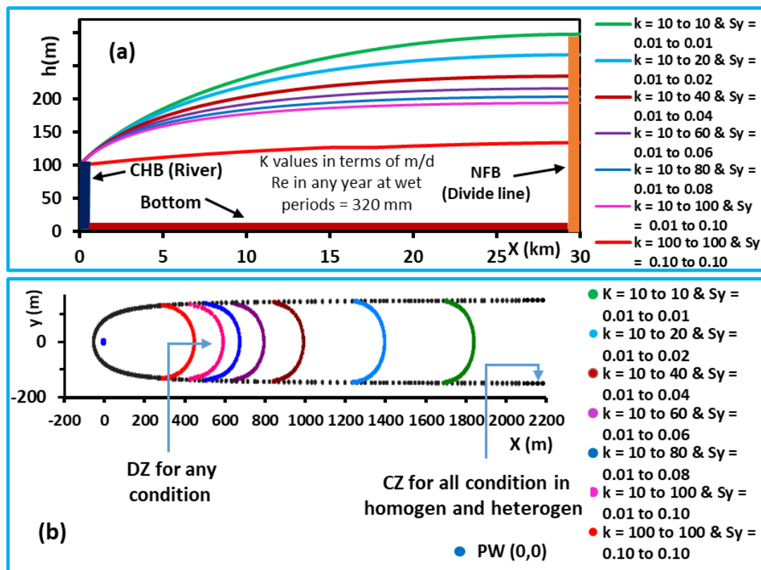
شکل ۹. اثر ناهمگنی: (a) سطح آب نرمال در پایان دوره‌ی تر. (b) حریم آبرگیر و حریم تخلیه. خطوط زمان گذر یک ساله هستند.
