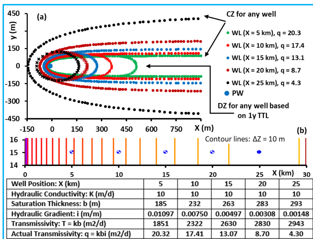
شکل ۱۳. (a) حریم آگیر و حریم تخلیه برای موقعیت چاه در جهت جریان از مرز تخلیه تا مرز تقسیم. (b) موقعیت چاه‌ها در عرض ۱۵ کیلومتری. خطوط زمان گذر ۱ ساله هستند.
