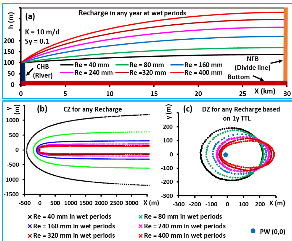
شکل ۱۰. اثر تغذیه سطحی ( Re ): (a) سطح آب نرمال در پایان دوره ی تر. (b) حریم آگیر. (c) حریم تخلیه. خطوط زمان گذر یک ساله هستند.
