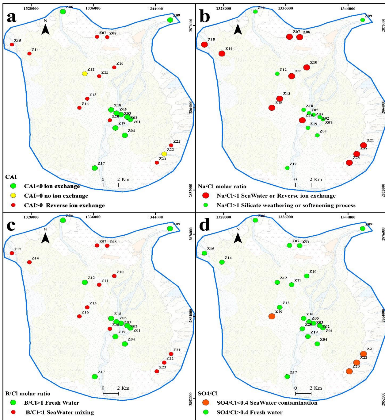
شکل ۹. توزیع مکانی نسبت‌های یونی (a) در مقابل \text{Cl}^- ، (b) \text{Na}^+/\text{Cl}^- ، (c) \text{B}/\text{Cl}^- و \text{SO}_4^{2-}/\text{Cl}^- نمونه‌های آب زیرزمینی در منطقه مورد مطالعه Fig. 9. Spatial distribution ionic ratios (a) CAI vs. \text{Cl}^- , (b) \text{Na}^+/\text{Cl}^- (c) \text{B}/\text{Cl}^- and (d) \text{SO}_4^{2-}/\text{Cl}^- groundwater samples in the study area
