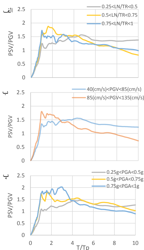
شکل ۶- طیف پاسخ شبه سرعت نرمال دوسویه با معیار پریود غالب T_p ، (با نماد (BNPVS(T_p)) )
