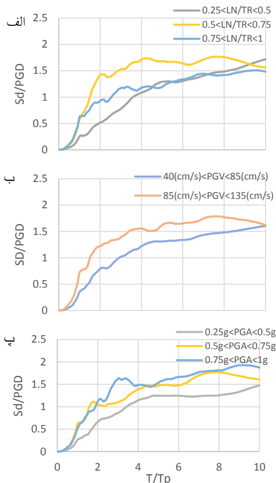
شکل ۵- طیف پاسخ جابجایی نرمال دوسویه با معیار پریود غالب T_p ، (با نماد (BND(S(T_p)) )
