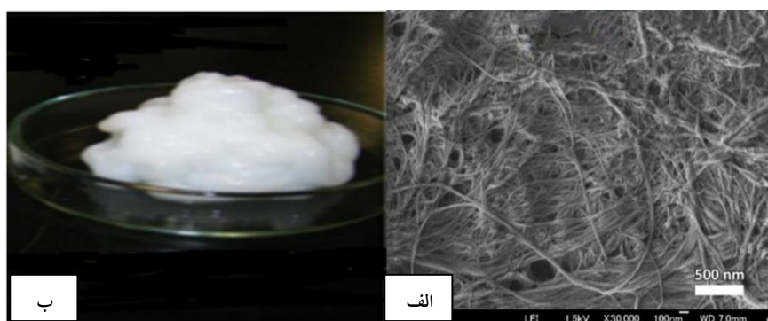
شکل ۳. الف) تصویر SEM نانو سلولز، ب) ژل نانو الیاف سلولز
