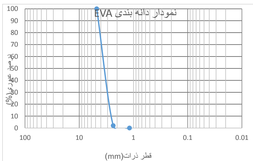
شکل ۴- منحنی دانه بندی EVA
