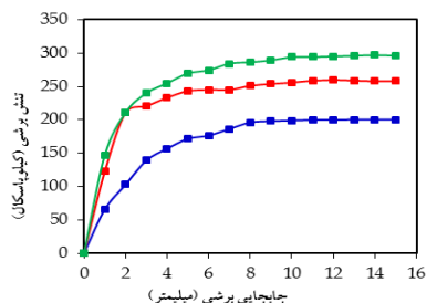
شکل ۱۱. آزمایش برش مستقیم نمونه بازسازی- شده در آزمایشگاه (بالا) و نمودار تنش- جابجایی برشی (پایین)
