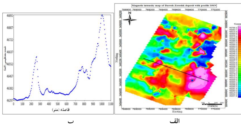
شکل ۹. الف) نقشه شدت میدان مغناطیسی کل همراه با موقعیت ایستگاه‌های برداشت مغناطیسی منطقه بر پروفیل ژئوالکتریکی 350N، ب) پروفیل بی‌هنجاری داده‌های ایستگاه‌های برداشت مغناطیسی منطقه بر پروفیل ژئوالکتریکی 350N
