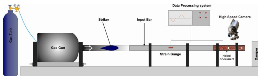
شکل ۲. اجزای آزمون میله فشاری‌هایکینسون اصلاح شده استفاده شده در این پژوهش
