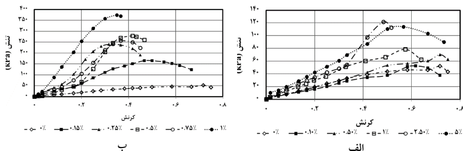
شکل ۷. تأثیر مقادیر مختلف نانوذرات بر مقاومت فشاری محصورنشده خاک بهسازی شده با (الف) نانورس (ب) نانوسیلیکا
