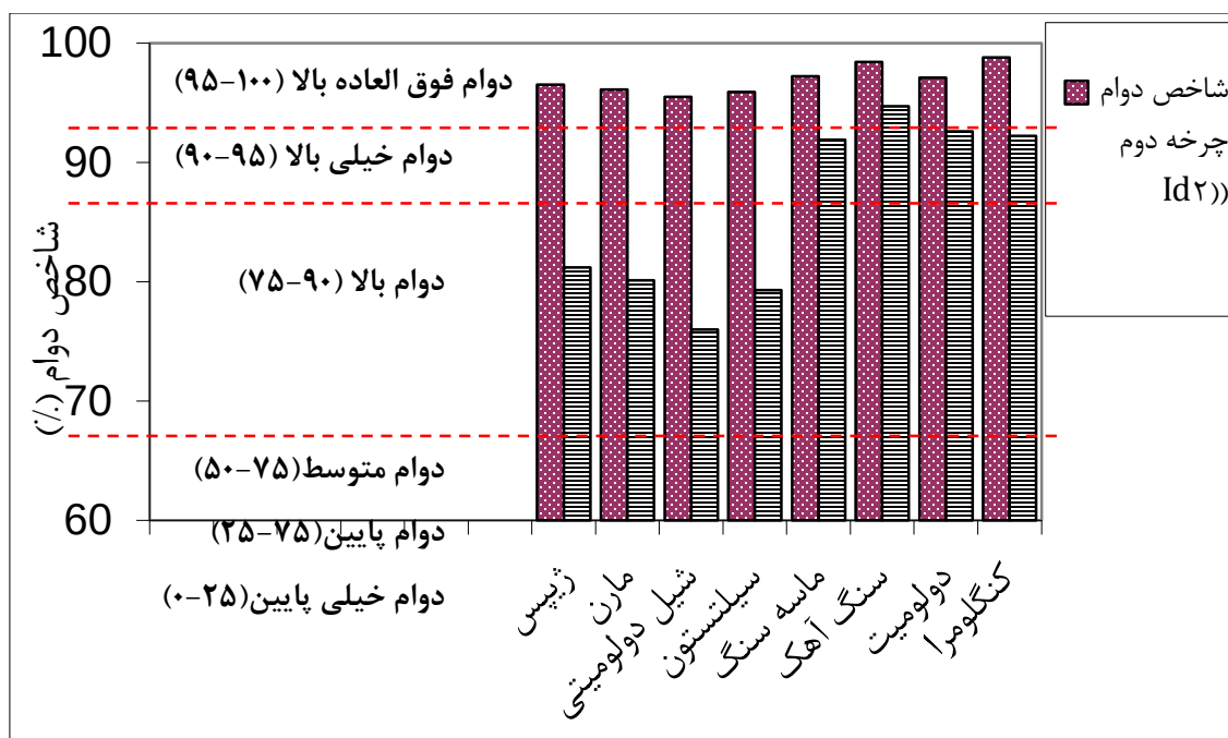
شکل ۷. طبقه بندی شاخص دوام نمونه‌ها در چرخه ۲ و ۱۵ آزمایش دوام وارفنگی در محلول نمک [۲۸]
