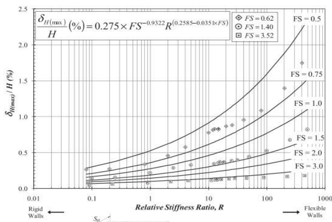
شکل ۱. تغییر شکل جانبی بر اساس سختی نسبی سیستم مهاری و ضریب اطمینان در برابر بالا آمدگی (بریسون و زاپاتا) [۲۰]
