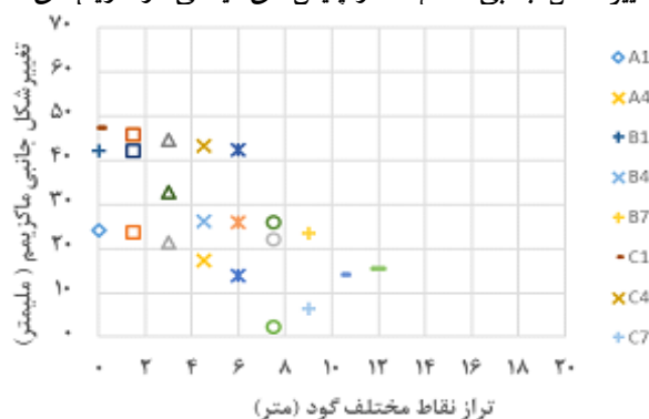
شکل ۹. تغییر شکل جانبی حداکثر برای نقاط داخل گود پس از اتمام عملیات حفاری
