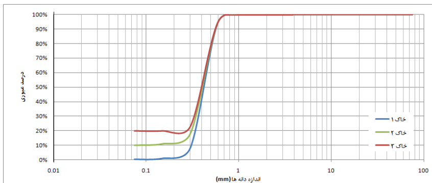
شکل ۱. دانه‌بندی خاک‌های آزمایش شده
