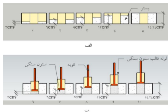
شکل ۱۲. مراحل انجام آزمایش‌ها در دستگاه برش مستقیم (الف) مراحل ساخت بستر، (ب) مراحل ساخت ستون سنگی
