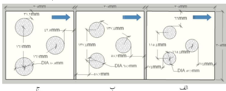
شکل ۱۰. آرایش قرارگیری ستون‌های سنگی در آرایش مربعی الف (۸/۴٪، ب) ۱۲٪، ج) ۱۶/۴٪، د) نمونه ساخته شده در دستگاه برش مستقیم
