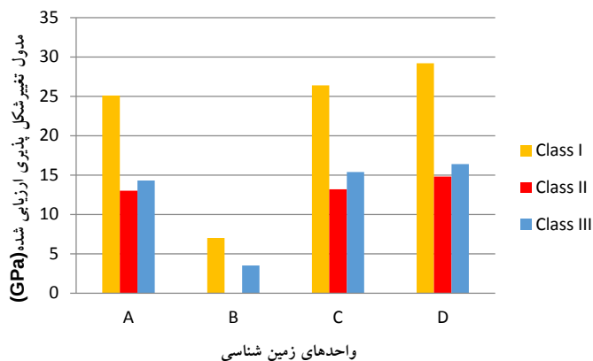
شکل ۲. مقایسهٔ مدول تغییر شکل پذیری ارزیابی شده به وسیلهٔ روش‌های تجربی در ساختمان سد بهشت‌آباد
