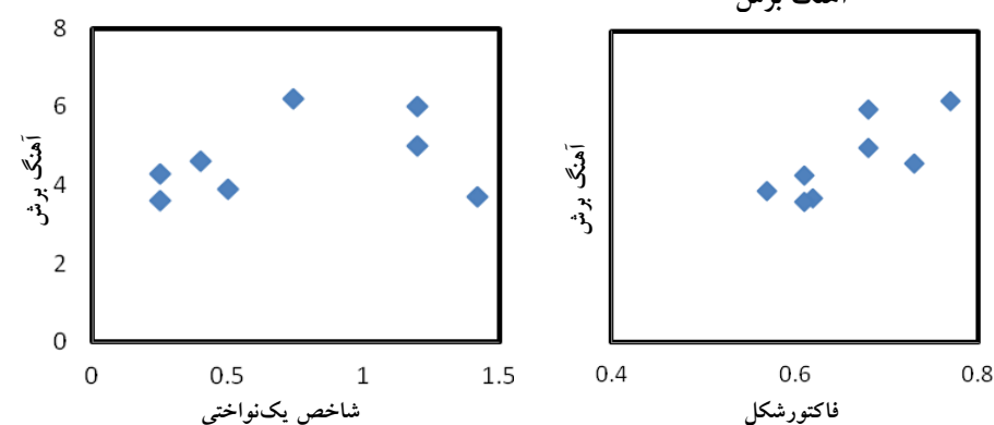
شکل ۹. ارتباط بین فاکتور شکل و آهنگ برش
