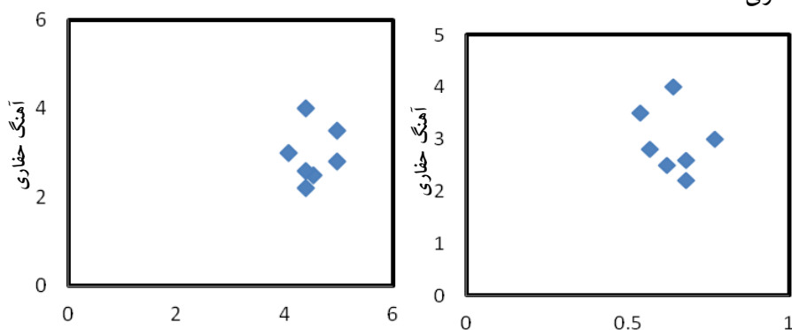
شکل ۱۹. ارتباط بین فاکتور شکل و آهنگ حفاری شکل ۲۰. ارتباط بین شاخص قفل‌شدگی و آهنگ حفاری
