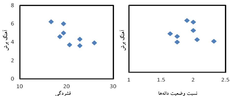
شکل ۷. ارتباط بین نسبت وضعیت دانه‌ها و آهنگ برش
