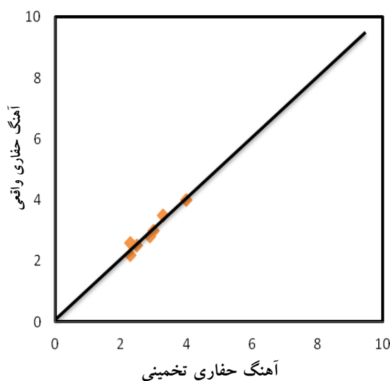
شکل ۲۲. مقایسه بین آهنگ حفاری واقعی و تخمینی
