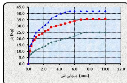
شکل ۷. نمودار بار-جایجایی افقی (خاک تثبیت شده با ۱٪ آهک و ۵٪ سرباره)
