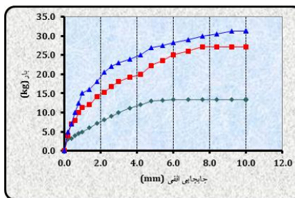
شکل ۲. نمودار بار-جایجایی افقی (خاک واگرا بدون افزودنی)
