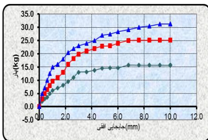
شکل ۳. نمودار بار-جایجایی افقی (خاک تثبیت شده با ۱٪ آهک)
