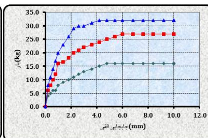
شکل ۴. نمودار بار-جایجایی افقی (خاک تثبیت شده با ۱٪ آهک و ۰/۵٪ سرباره)
