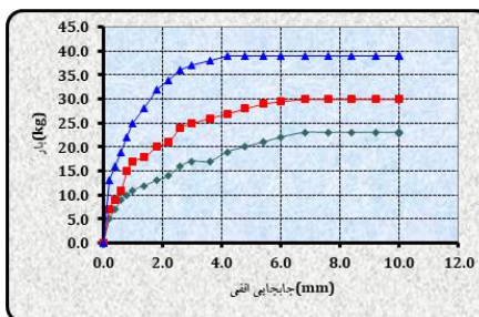
شکل ۶. نمودار بار-جایجایی افقی (خاک تثبیت شده با ۱٪ آهک و ۳٪ سرباره)
