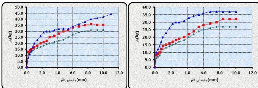
شکل ۸. نمودار بار-جابجایی افقی خاک تثبیت شده با ۲٪ آهک و ۰٫۵٪ سرباره) شکل ۹. نمودار بار-جابجایی افقی خاک تثبیت شده با ۲٪ آهک و ۱٪ سرباره)
