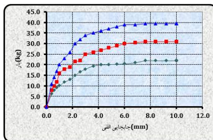
شکل ۵. نمودار بار-جایجایی افقی (خاک تثبیت شده با ۱٪ آهک و ۱٪ سرباره)
