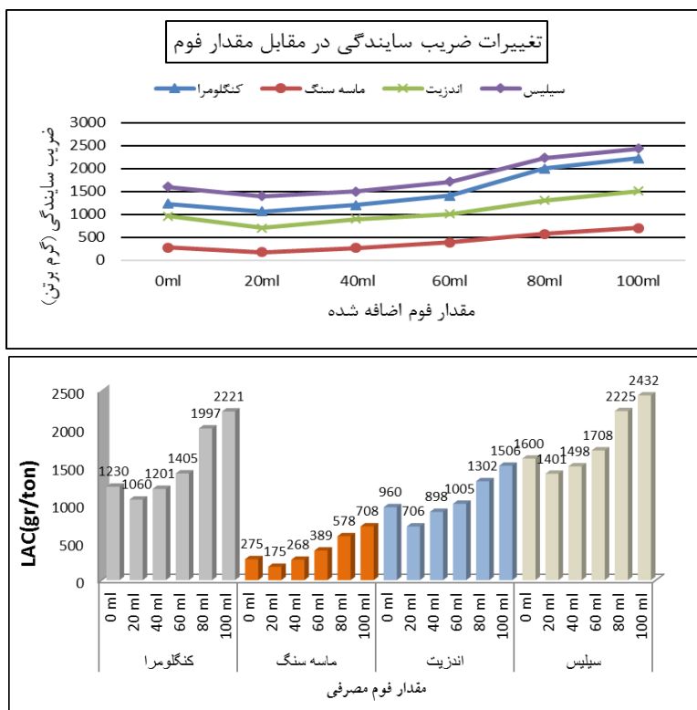
شکل ۱۳. نتایج آزمایش تعیین ساینده‌گی مصالح فوم دار به کمک دستگاه LCPC
