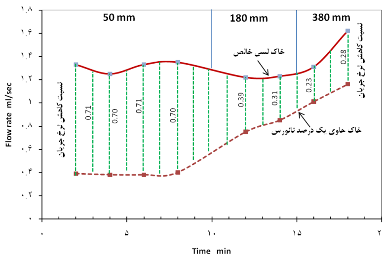
شکل ۱۹. تغییرات نسبت کاهش جریان در اختلاط به‌روش D با افزودن ۱ درصد نانورس
