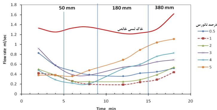
شکل ۱۲. نتایج تغییرات نرخ جریان در آزمایش پین‌هول بر روی اختلاط خاک لس مراوه تپه با نانورس به روش تهیه گل همگن به وسیله هم‌زن برقی (روش A)
