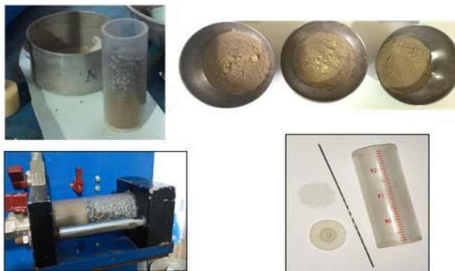
شکل ۵. مراحل آماده‌سازی و انجام آزمایش در دستگاه پین‌هول
