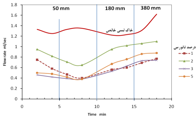
شکل ۱۳. نتایج تغییرات نرخ جریان در آزمایش پین‌هول بر روی اختلاط خاک لسی مراوه تپه با نانورس در رطوبت بهینه به وسیله ورزدادن با دست (روش B)
