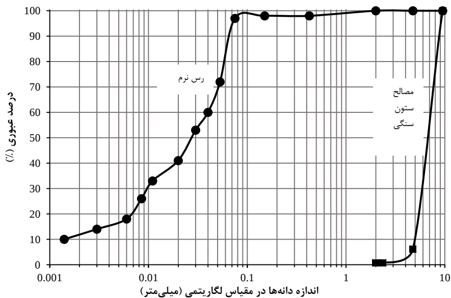
شکل ۲. نمودار دانه‌بندی خاک رس و مصلح ستون سنگی
