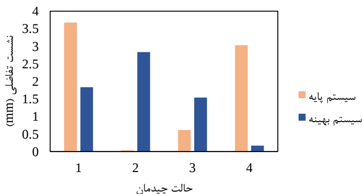
شکل ۱۸. مقایسه نمودار نشست تفاضلی سیستم مرکب پی - شمع بهینه (با طول شمع‌های متغیر) و سیستم پایه (آرایش یک‌نواخت) بر خاک دانه‌ای
