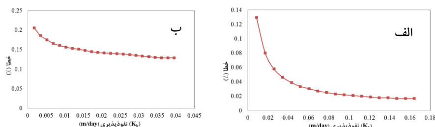
شکل ۱۹. الف) نمودار کمیته‌سازی تابع خطا برای پارامتر K_h در لایه‌های ML ناحیه ۲ ژئوتکنیکی در محل خاکریز EM-3، ب) نمودار کمیته‌سازی تابع خطا برای پارامتر K_h در لایه‌های CL-2 ناحیه ۲ ژئوتکنیکی در محل خاکریز EM-3
