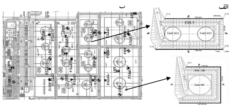
شکل ۷. الف) پلان موقعیت خاکریزهای EM-3 و EM-2B، ب) محل گمانه های ناحیه دو و سه ژئوتکنیکی
