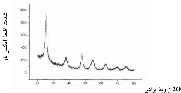
شکل ۵. پراش XRD نمونه نانو مواد کربنات کلسیم
