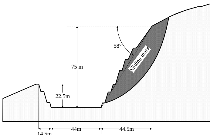
شکل ۶. تحلیل پایداری شيروانی جناح راست سرریز برای شرایط استاتیکی
