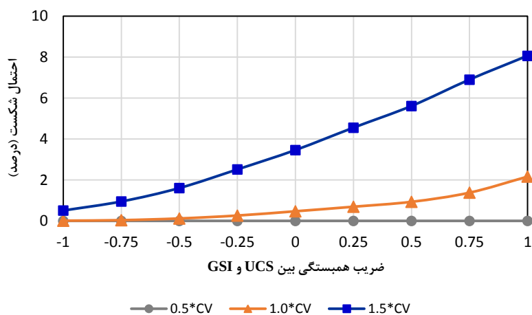
شکل ۱۷. توزیع احتمال ضریب اطمینان استاتیکی شیروانی جناح راست سرریز به‌ازای ضریب تغییرات مختلف کمیت‌ها برای حالت بعد از باربرداری
