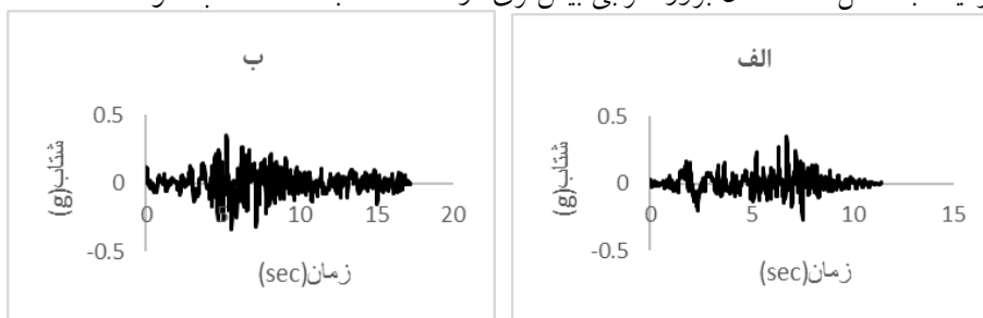
شکل ۲. تاریخچه رکورد شتاب نرمالیزه شده با شتاب ۰/۳g. برای زلزله‌های الف) سان فرناندو، ب) طبس
