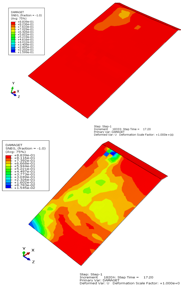
شکل ۱۰. مقایسه خرابی روکش بتنی تحت زلزله طبس در سه حالت؛ الف) خالی، ب) نیمه پر و ج) پر
