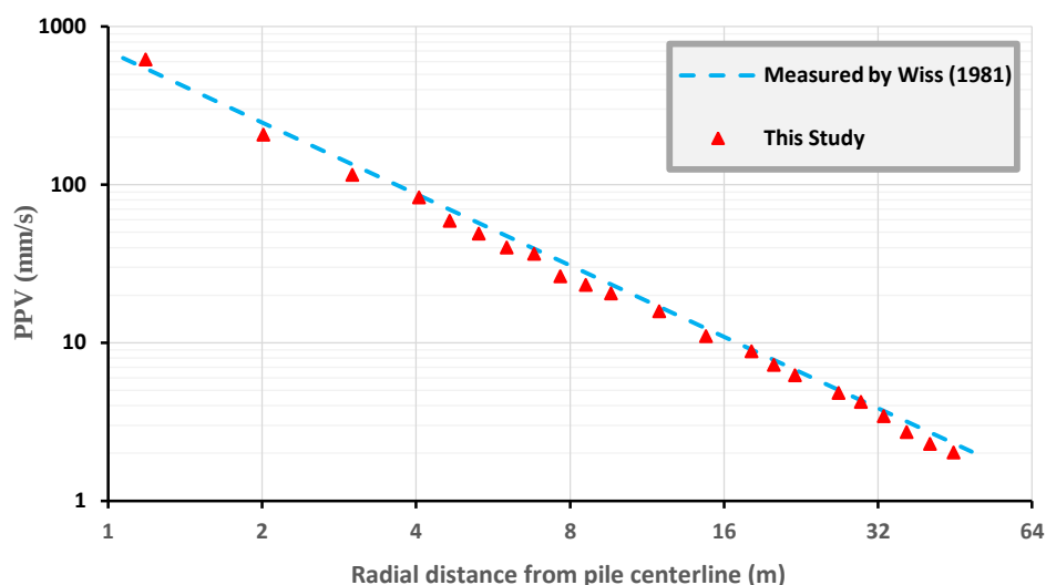
شکل ۷. مقایسه حداکثر سرعت ذره حاصل از مدل‌سازی عددی با نتایج صحرایی ویس (1981) برای ذرات در سطح زمین با فواصل افقی مختلف در عملیات شمع‌کوبی ضربه‌ای
