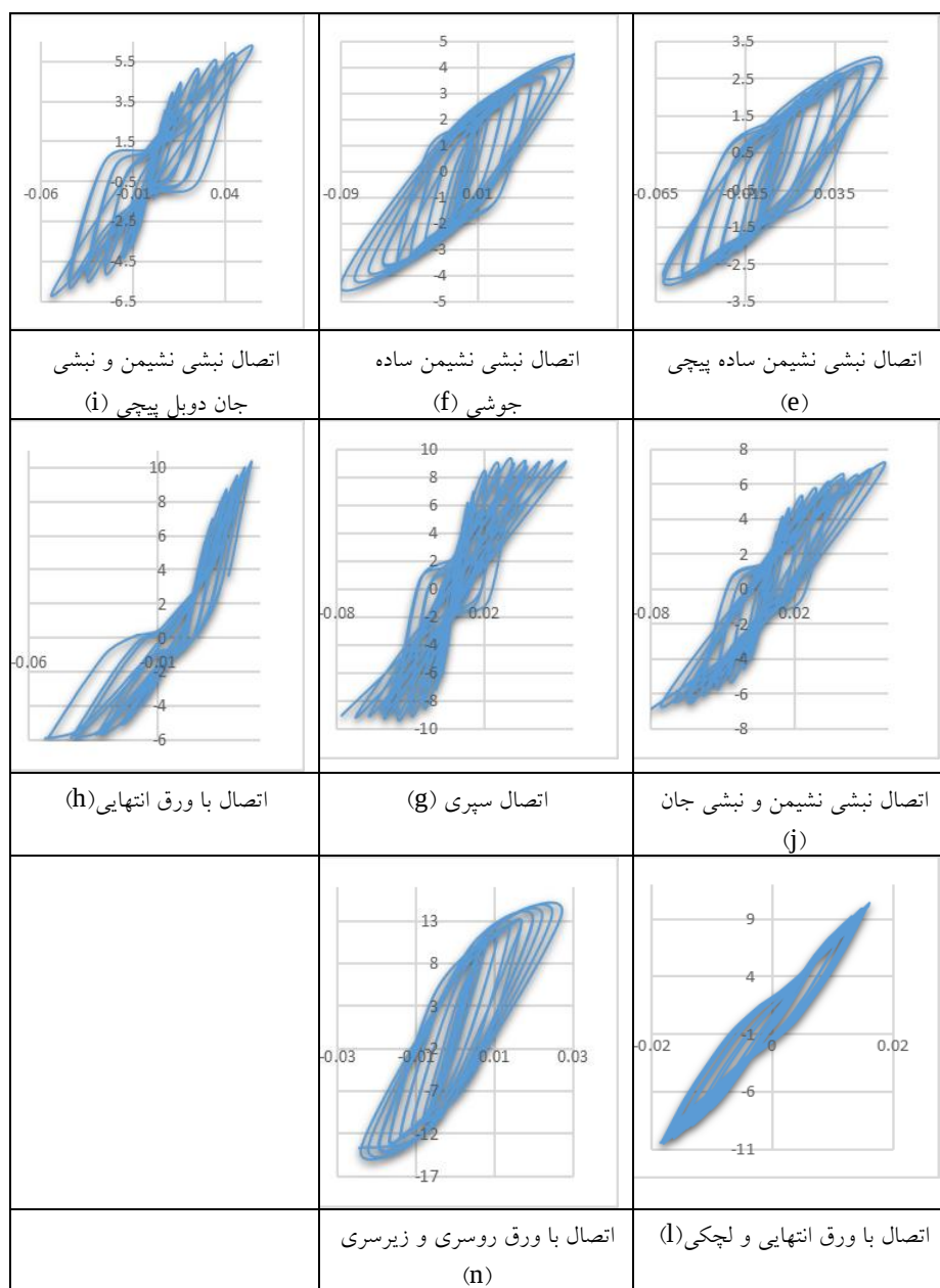
شکل ۱۵. منحنی لنگر چرخش اتصالات نیمه صلب رایج
