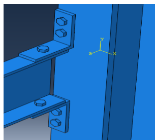
شکل ۴. اتصال نبشی نشیمن ساده پیچی (e)
