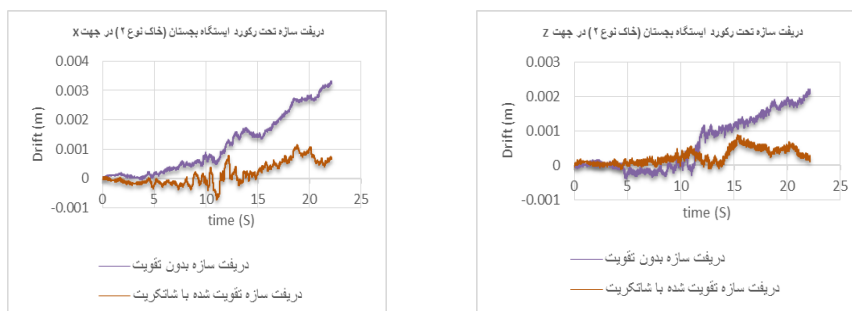
شکل ۲۰. دررفت سازه تحت رکورد ایستگاه بجستان (خاک نوع II)
