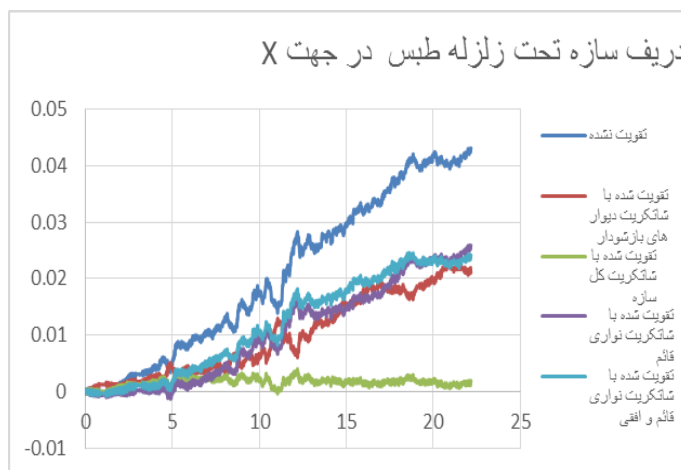
شکل ۱۲. ب) نمودار دررفت سازه تحت زلزله طیس در جهت X
