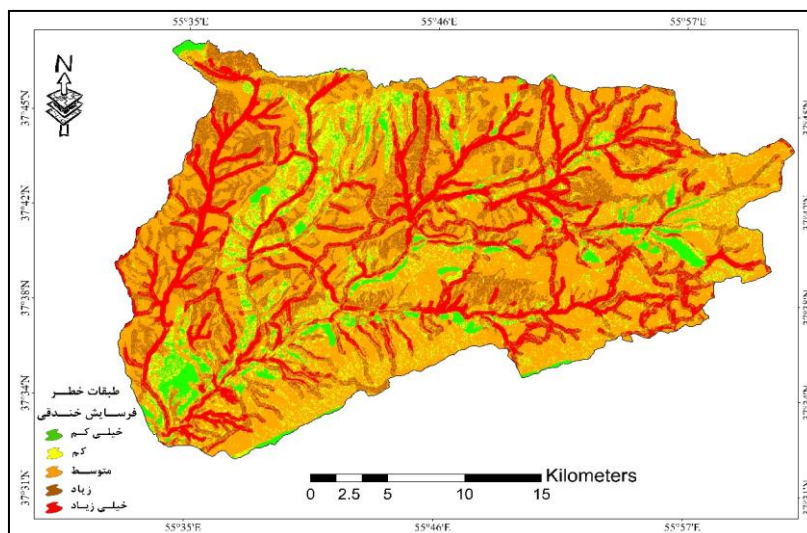
شکل ۵. نقشه پهنه‌بندی خطر فرسایش خندقی حوزه آبخیز قرناوه با استفاده از مدل GNR ۴. مساحت و درصد طبقات خطر فرسایش خندقی در حوزه آبخیز قرناوه با استفاده از مدل نسبت فراوانی و GNR
