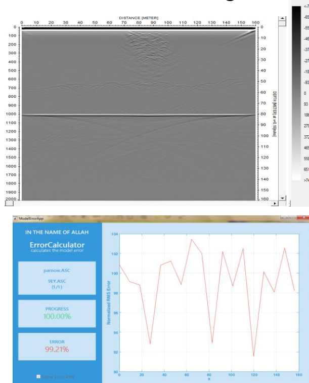
شکل ۹. مدل زمین با بیش‌ترین شباهت به مقطع حاصل از برداشت داده‌های صحرایی در منطقه یخچال علم‌کوه همراه با میزان خطای به‌دست آمده
