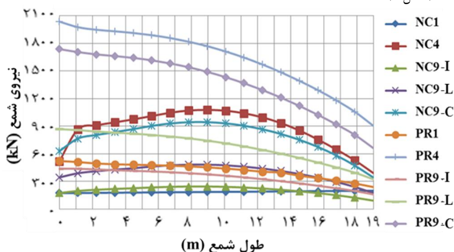
شکل ۶. منحنی تغییرات نیروی شمع‌ها بر حسب طول آن در حالت‌های مختلف (نماد PR و NC به ترتیب به معنای شمع متصل و غیرمتصل و اعداد بعد از آن نشان‌دهنده تعداد شمع است)
