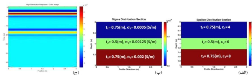
شکل ۴. الف) مقطع توزیع گذردهی دی‌الکتریک، ب) مقطع توزیع هدایت الکتریکی و ج) پاسخ GPR یک مدل زمین سه‌لایه‌ای که هر سه لایه، آهکی هستند ( \sigma هدایت الکتریکی برحسب زیمنس بر متر و t ضخامت لایه بر حسب متر است).
