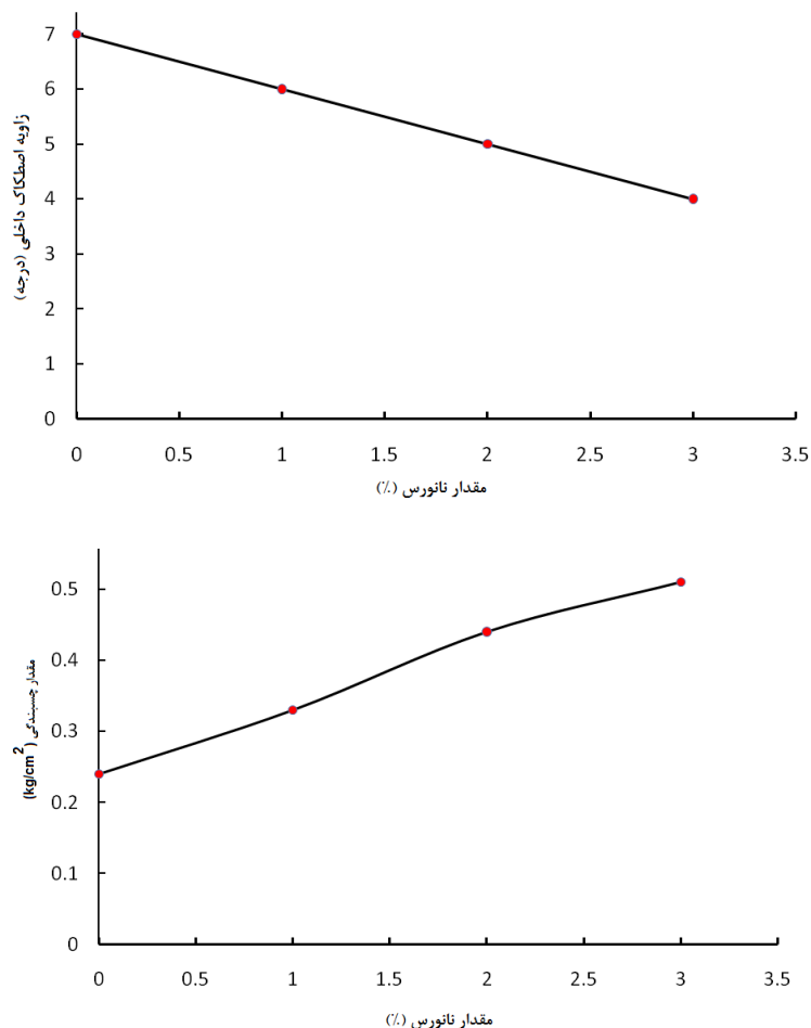
شکل ۹. تأثیر افزودن نانورس بر پارامترهای مقاومت برشی نمونه‌ها در شبکه سد بوستان گنبد
