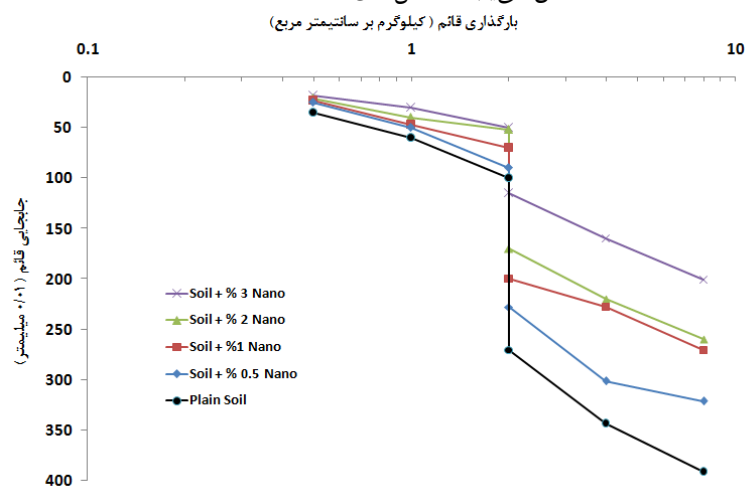
شکل ۱۰. تأثیر افزودن نانورس بر مشخصات تحکیمی نمونه‌های خاک شبکه سد بوستان گنبد
