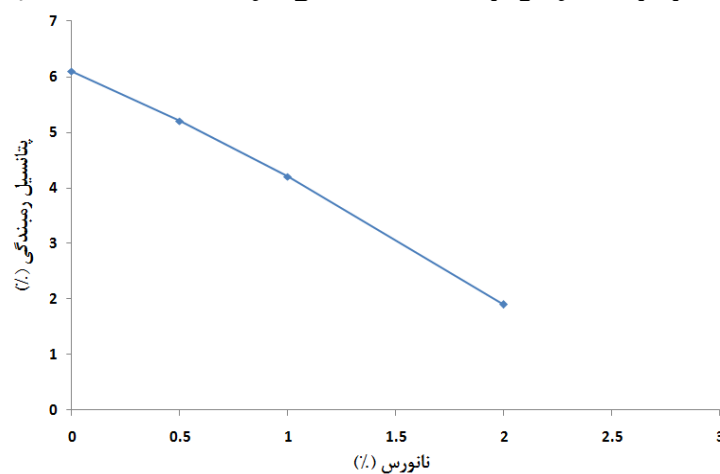
شکل ۱۱. تأثیر افزودن نانورس بر پتانسیل رمبندگی نمونه‌های خاک شبکه سد بوستان گنبد
