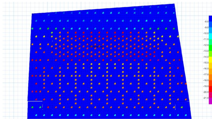
شکل ۱۴. پلان جانمایی نهایی ستون‌های جت‌گروتینگ در طرح اصلاح شده ( \text{kg/cm}^2 )
