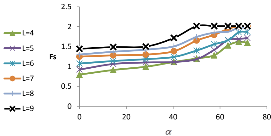
شکل ۵. تغییرات ضریب اطمینان در برابر چیدمان میخ
