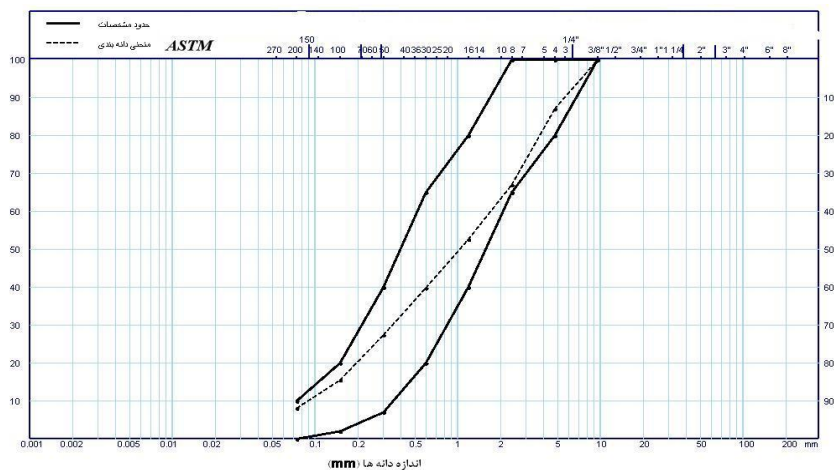
نمودار ۳. دانه‌بندی ماسه شکسته (۶-۲۰) میلی‌متر
