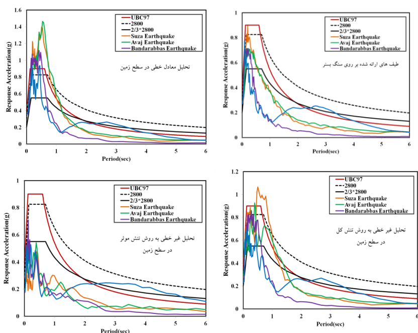
۱۰. مقایسه شتاب‌های طیف تحلیل پاسخ زمین به روش معادل خطی، غیرخطی (تنش کل، تنش مؤثر) و طیف طراحی پاسخ ارائه شده در آیین‌نامه‌های ۲۸۰۰ و UBC97
