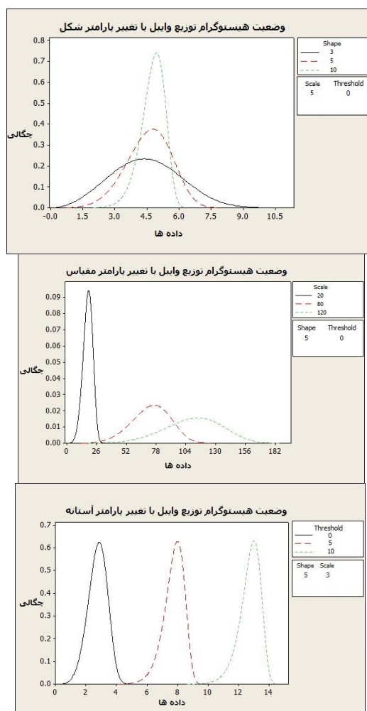
شکل ۴. تغییر وضعیت توزیع وایل با تغییر پارامترهای توزیع
