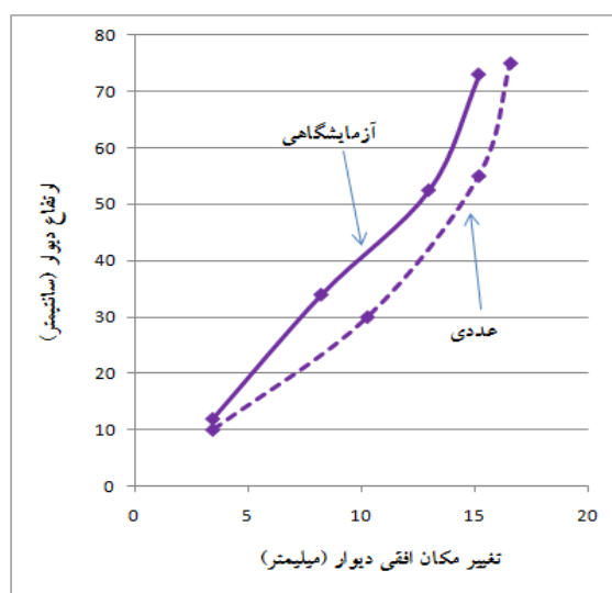
شکل ۴. مقایسه نتایج مدل‌سازی فیزیکی و آزمایشگاهی در دیوار 5-p-wa5
