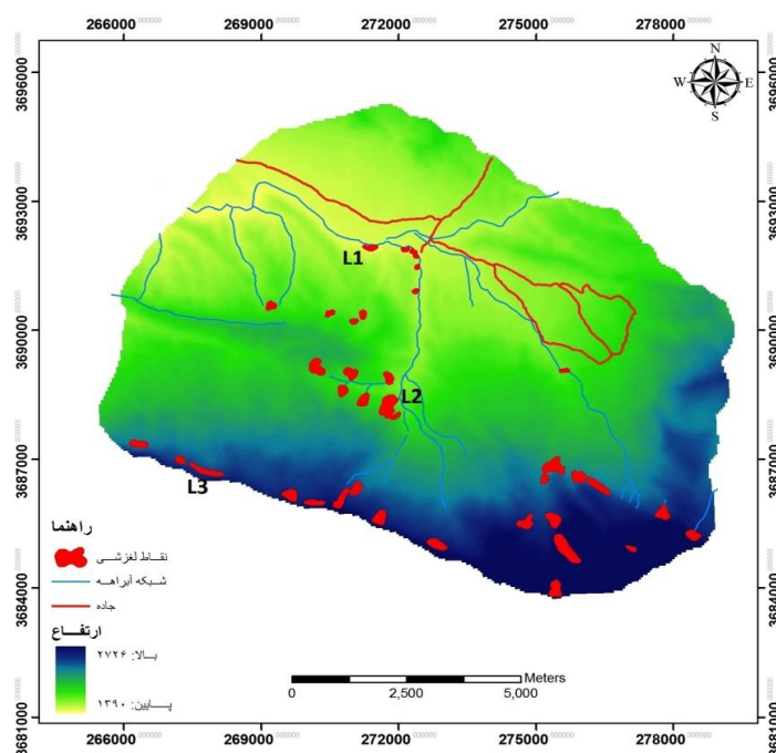
شکل ۲. نقشه پراکنش زمین‌لغزش در حوضه کاکاشرف
