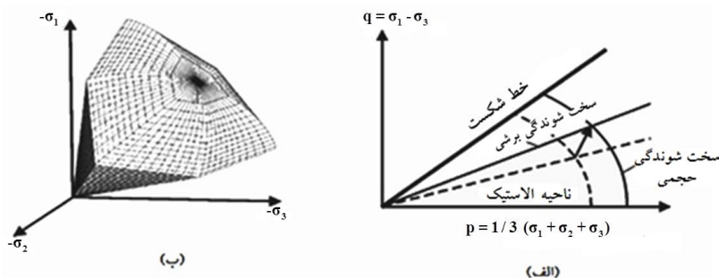
شکل ۶. سطح تسلیم برای مدل خاک سخت شونده در C=0 الف) سخت شونده گی برشی و حجیمی در فضای p-q ، ب) سطح تسلیم کل در فضای تنش‌های اصلی [۳۱]
