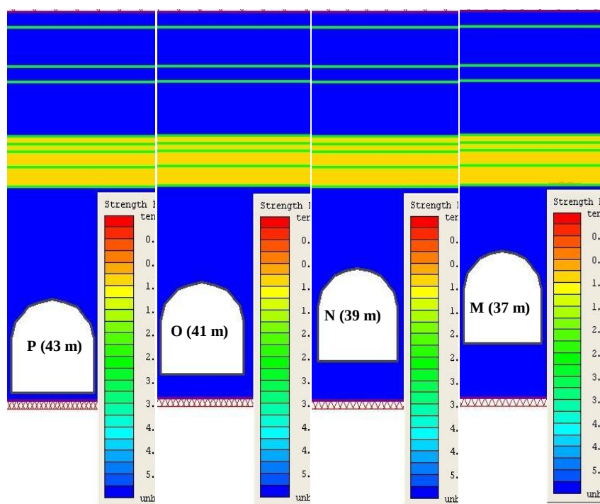
ادامه شکل ۶. آنالیز گسترش مقادیر ضریب ایمنی از عمق ۱۳ الی ۴۳ متری
