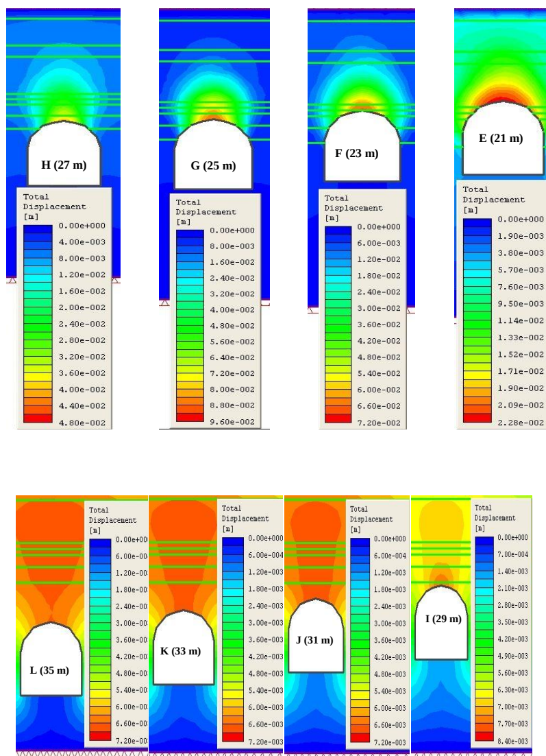
ادامه شکل ۵. نتایج آنالیز عددی میزان جابه‌جایی الاستیک از عمق ۱۳ الی ۴۳ متری.
