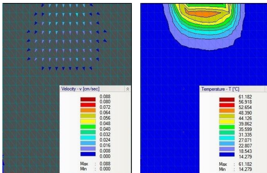
شکل ۱۲. الف) محیط مدل‌سازی شده به همراه کنتورهای حرارتی و ب) بردارهای سرعت نفوذ آب تزریقی
