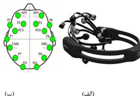
شکل ۲. (الف) هدست Emotive EPOC+، (ب) نحوه قرار گرفتن الکترودها روی سر
