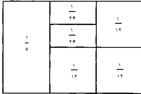
شکل ۳. نشان‌دادن حاصل‌جمع \frac{1}{6} + \frac{3}{12} + \frac{2}{24}
